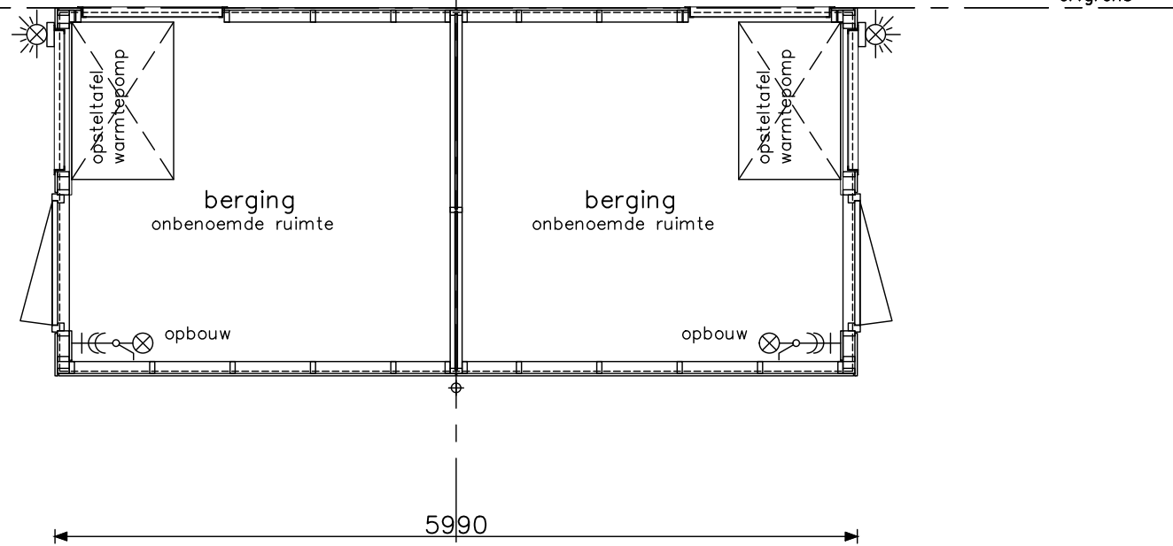
plattegrond
